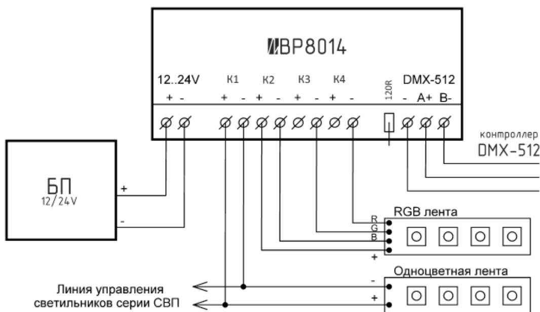
Принципиальная схема подключения.
