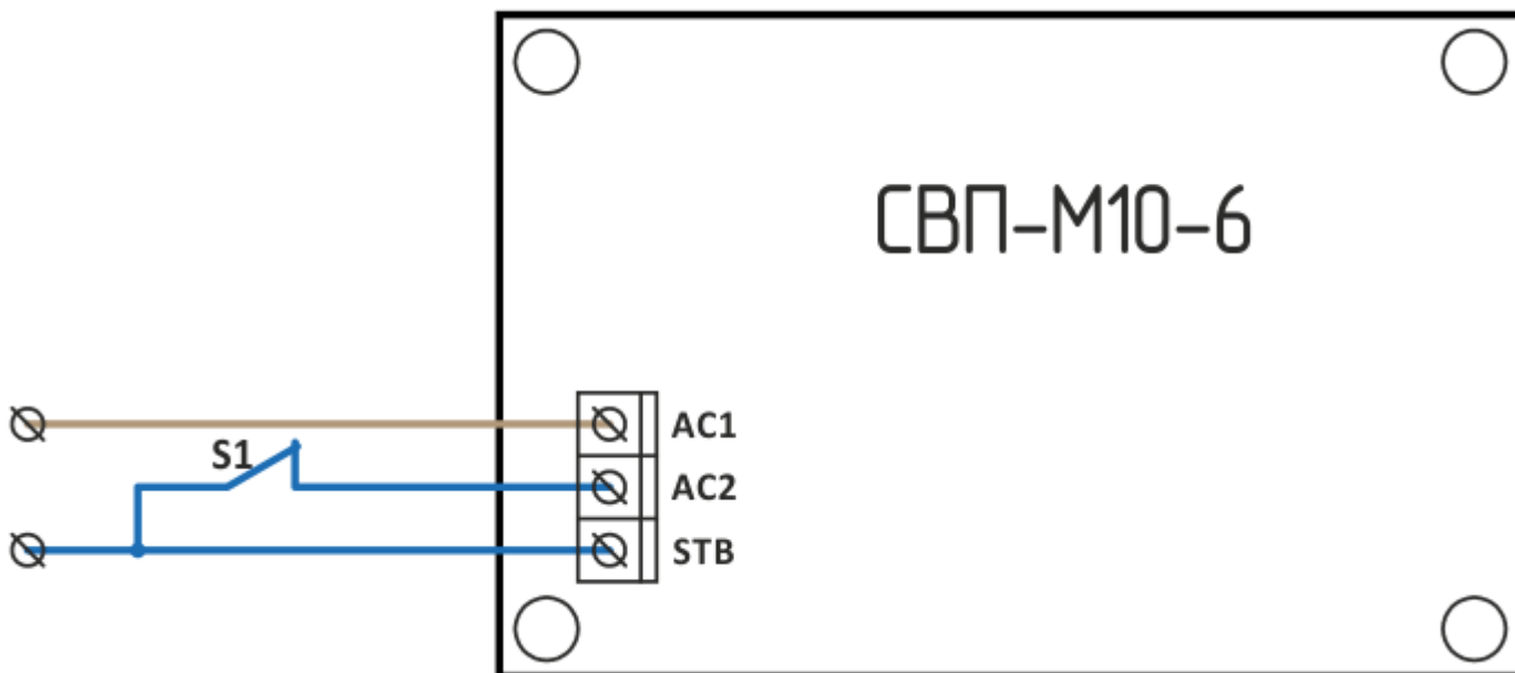
схема подключения модуля СВП-М13-7
